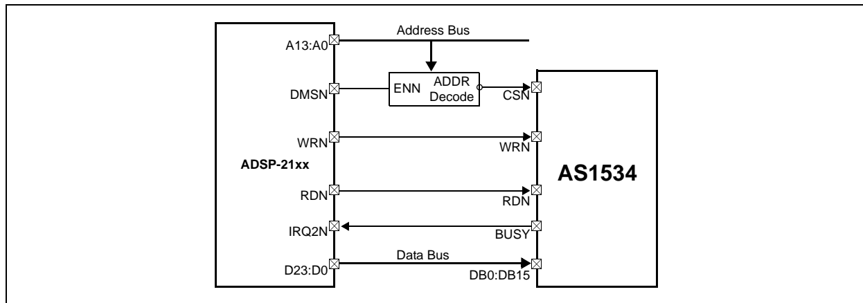
Figure 28. ADSP-21xx Interface
